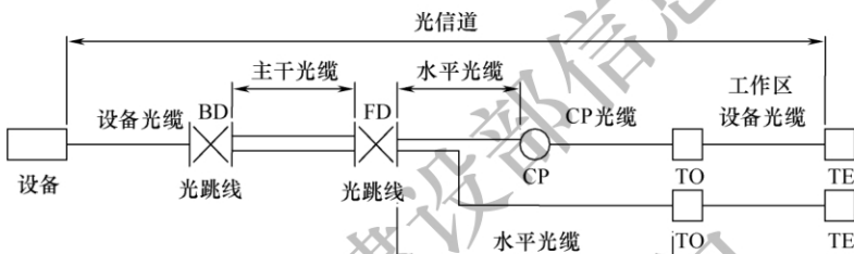
图 3.2.4-1 光纤信道构成 1
