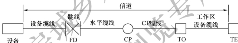
图 3.3.2 配线子系统缆线划分
