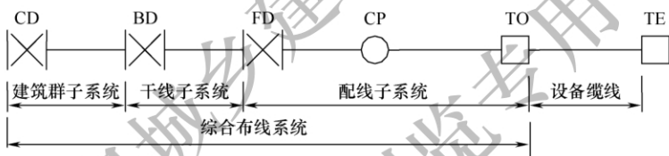
图 3.1.2-1 综合布线系统基本构成
