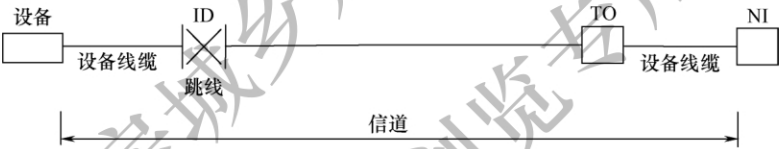
图 3.7.8 中间配线子系统构成
