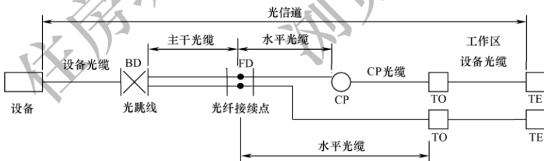
图 3.2.4-2 光纤信道构成 2
