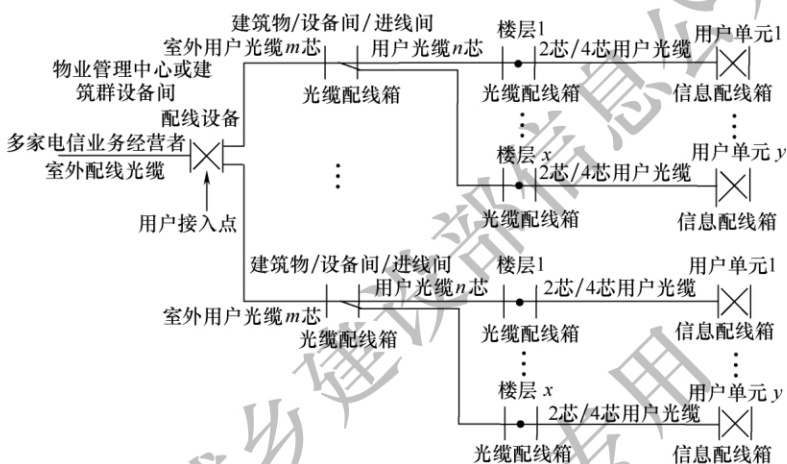
图 4.2.2-3 用户接入点设于建筑群物业管理中心机房或综合布线设备间或通信机房
