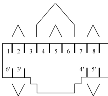
图 6.1.3-2 7 类和 7 A 类模块插座连接(正视)方式 1
