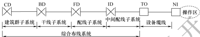
图 3.7.3 工业环境布线系统架构
