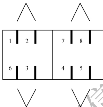
图 6.1.3-3 7 类和 7 A 类插座连接(正视)方式 2
