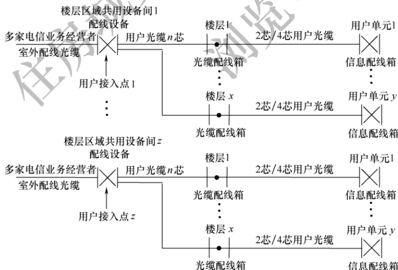
图 4.2.2-2 用户接入点设于建筑物楼层区域共用设备间
