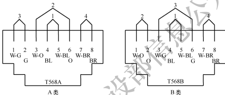
图 6.1.3-1 8 位模块式通用插座连接
