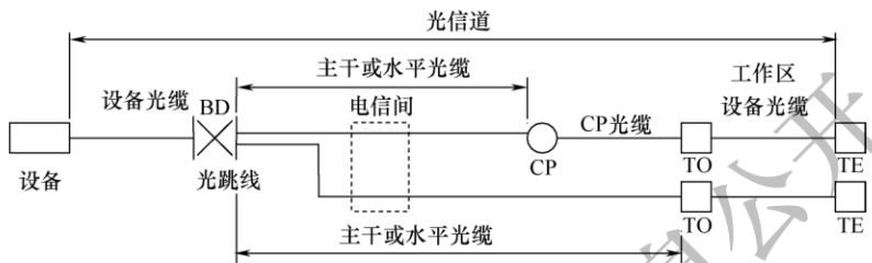
图 3.2.4-3 光纤信道构成 3
