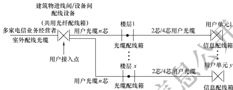
图 4.2.2-4 用户接入点设于进线间或综合布线设备间或通信机房
