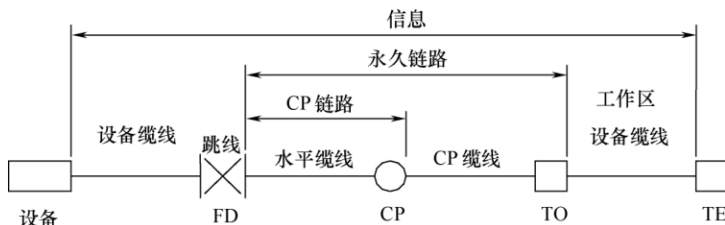
图 3.2.2 布线系统信道、永久链路、CP 链路构成
