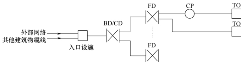
图 3.1.1.2-3 综合布线系统引入部分构成
