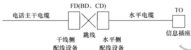
图 5.2.3-1 电话交换系统中缆线与配线设备间连接方式
