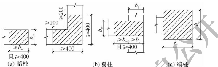
图 6.4.5-1 抗震墙的构造边缘构件范围
