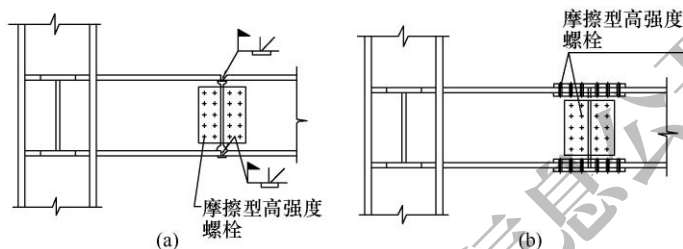
图 8.3.4-2 框架柱与梁悬臂段的连接
